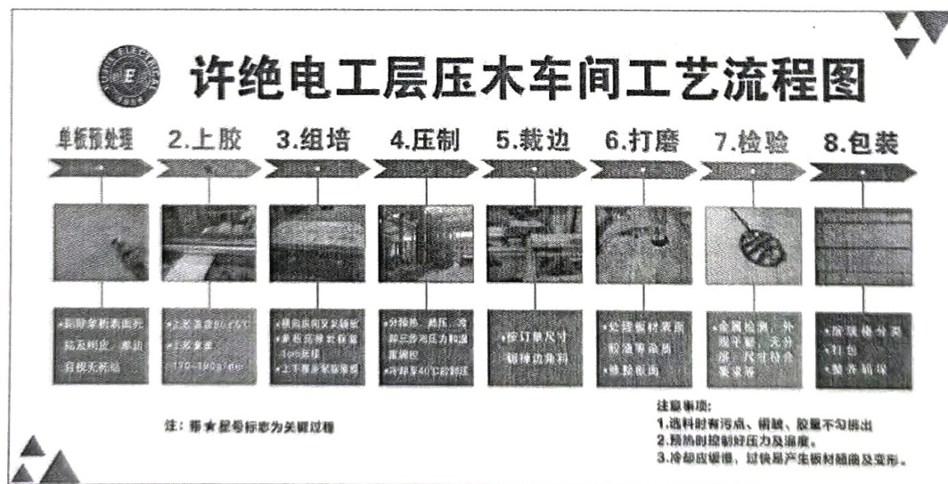
图 2.2 压木车间工艺流程图
